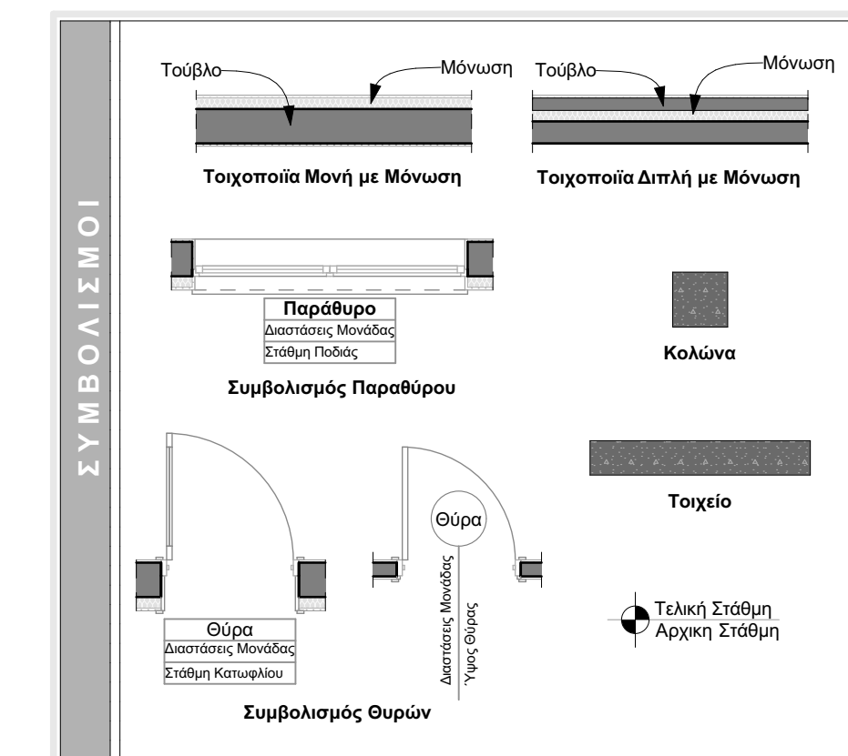
S-01 ΣΥΜΒΟΛΙΣΜΟΙ 1:50
