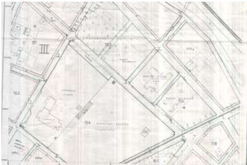
Απόσπασμα πινακίδας Π_2.1 (8.08) Πολεοδομική μελέτη Προσοτσάνης
